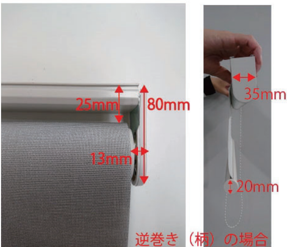
(メカ部寸法参考)
