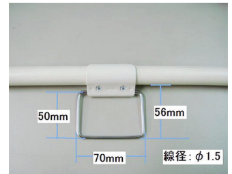
(プルハンドル寸法参考)
